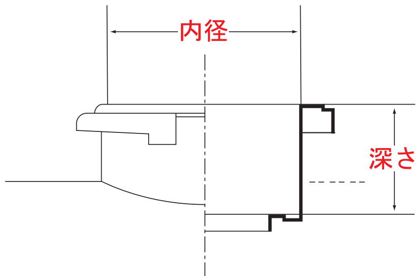
現車フィラーネック(つめ式)
